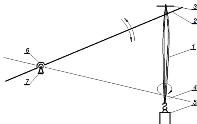
Зураг 1. Уламжлалт аргаар сур элдэх машины технологийн бүдүүвч
